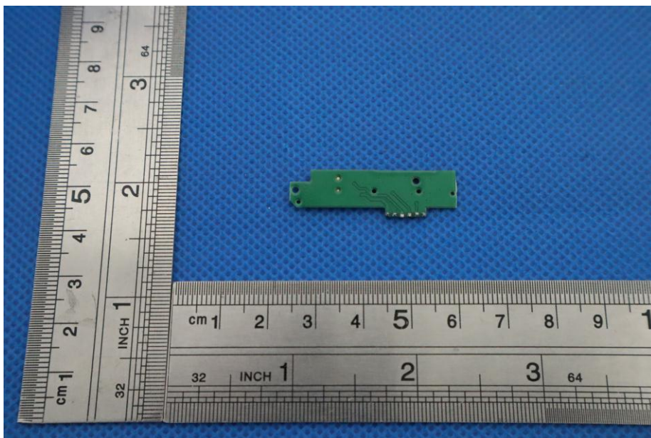
EUT Photo 8
