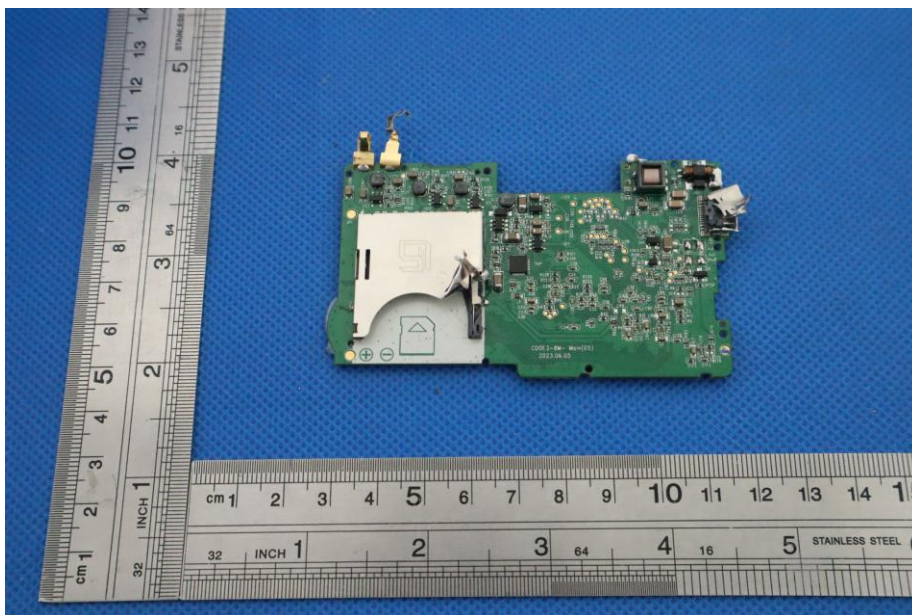
EUT Photo 6
